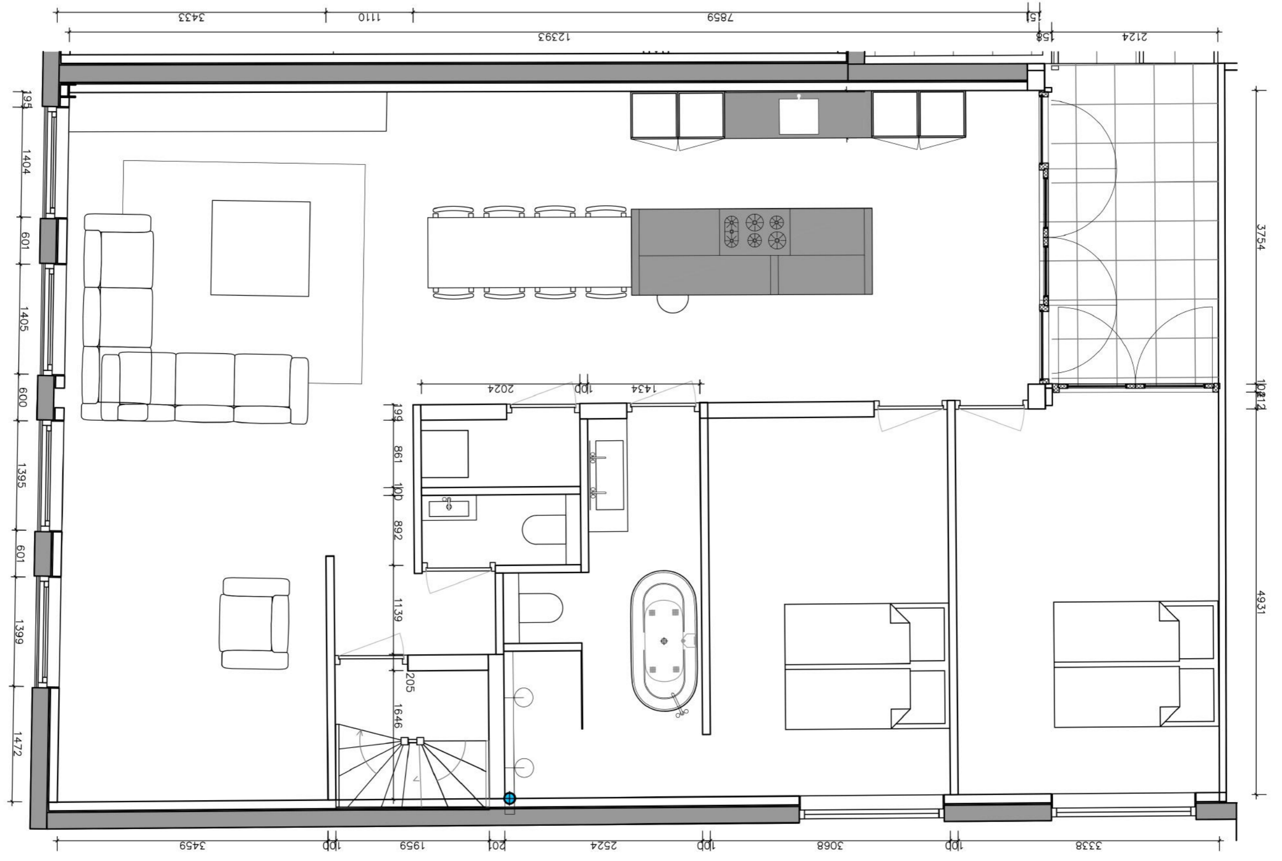
NUMMER 2 eerste verdieping
